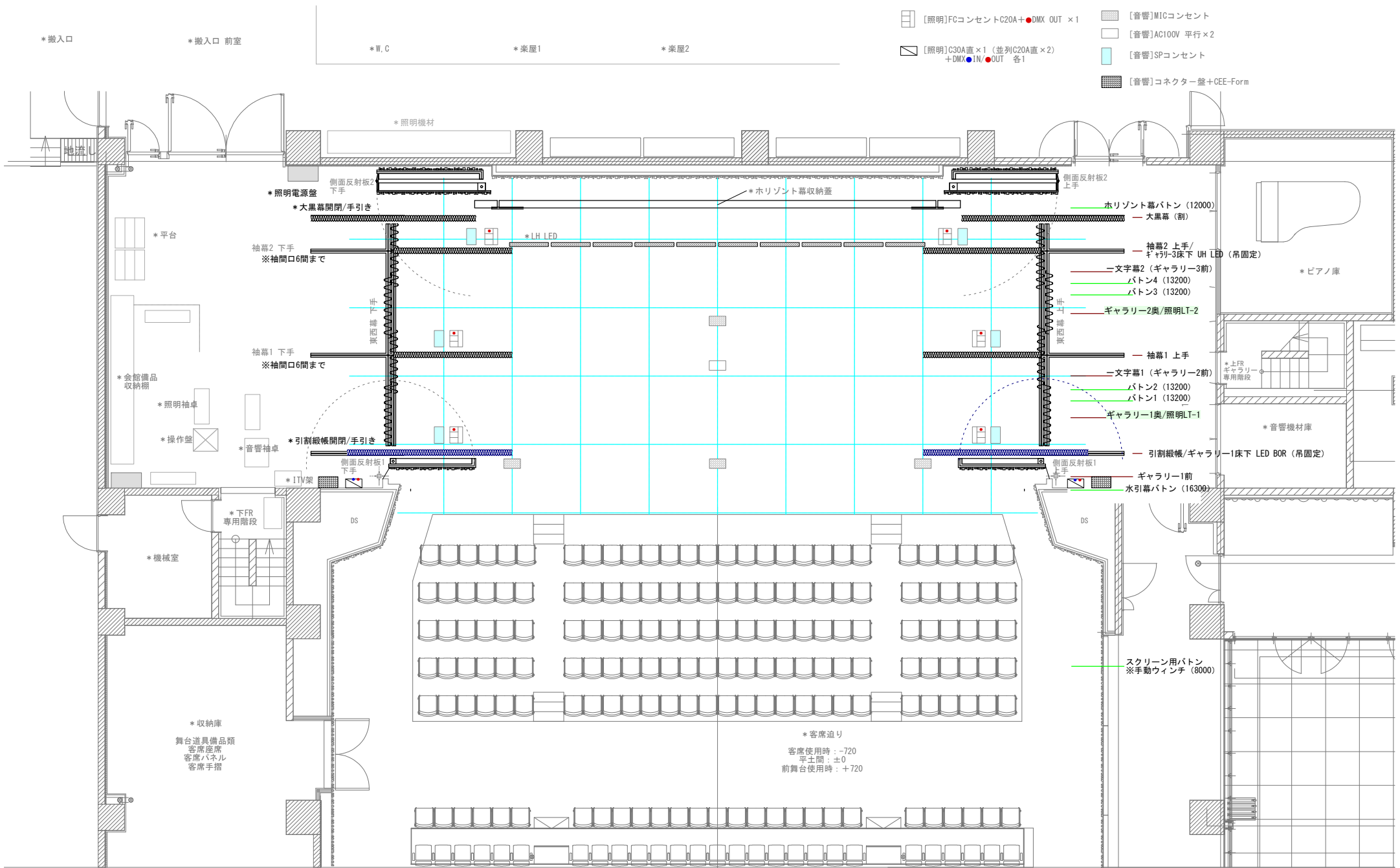
邑楽町中央公民館 ホール 舞台平面図
